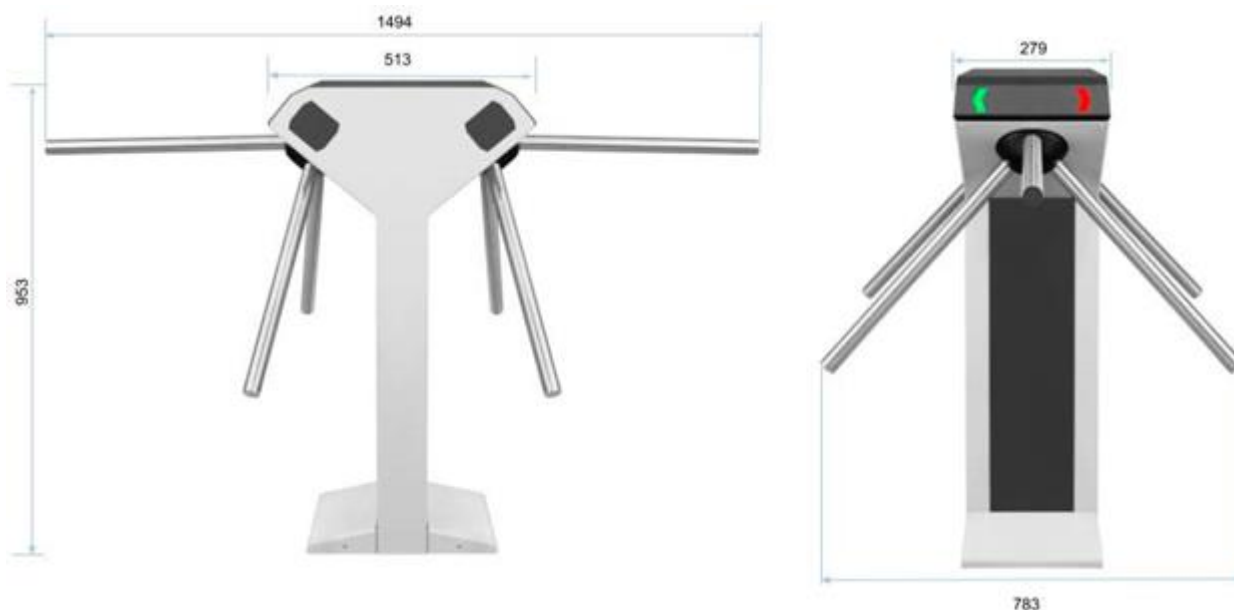
Рисунок 5.1 - Габаритные размеры турникета с планками «ТDХ-01»
